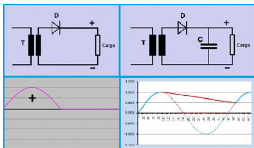
Figura 1- Fuente monofásica de media onda
