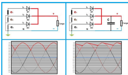
Figura 3- Fuente trifásica de media onda
