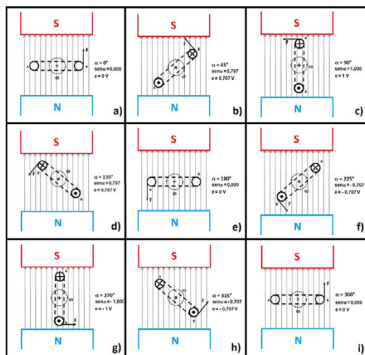
Figura 2- Fuerza electromotriz inducida según la posición de la bobina
