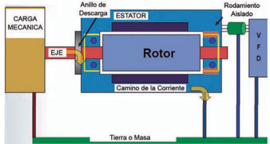
Figura 5. Solución con Anillo de Descarga y Rodamiento Aislado.
