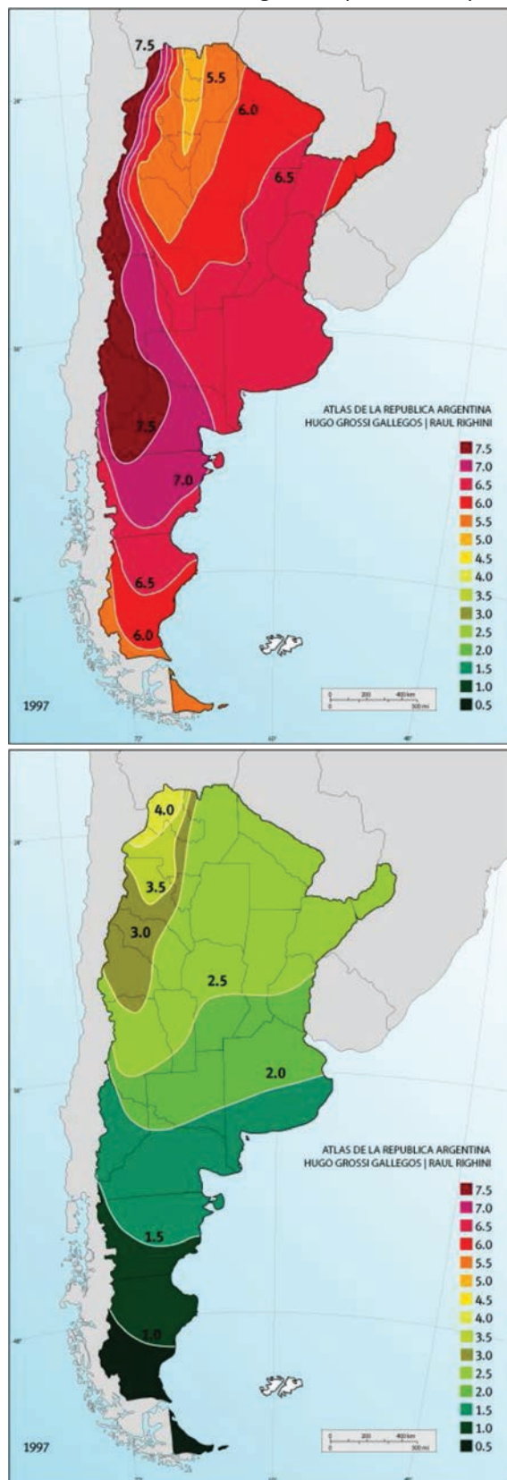
Figura 25. Mapas de radiación solar en Argentina en enero (arriba) y julio (abajo) en kWh/m 2 . Fuente: Atlas de Energía Solar de Argentina Continuará...
